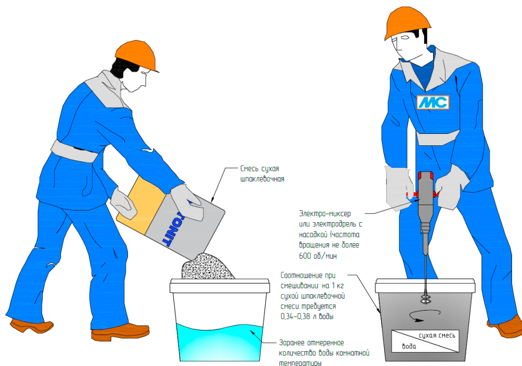
Рис. 9. Организация работ по затворению сухой шпаклевочной смеси
